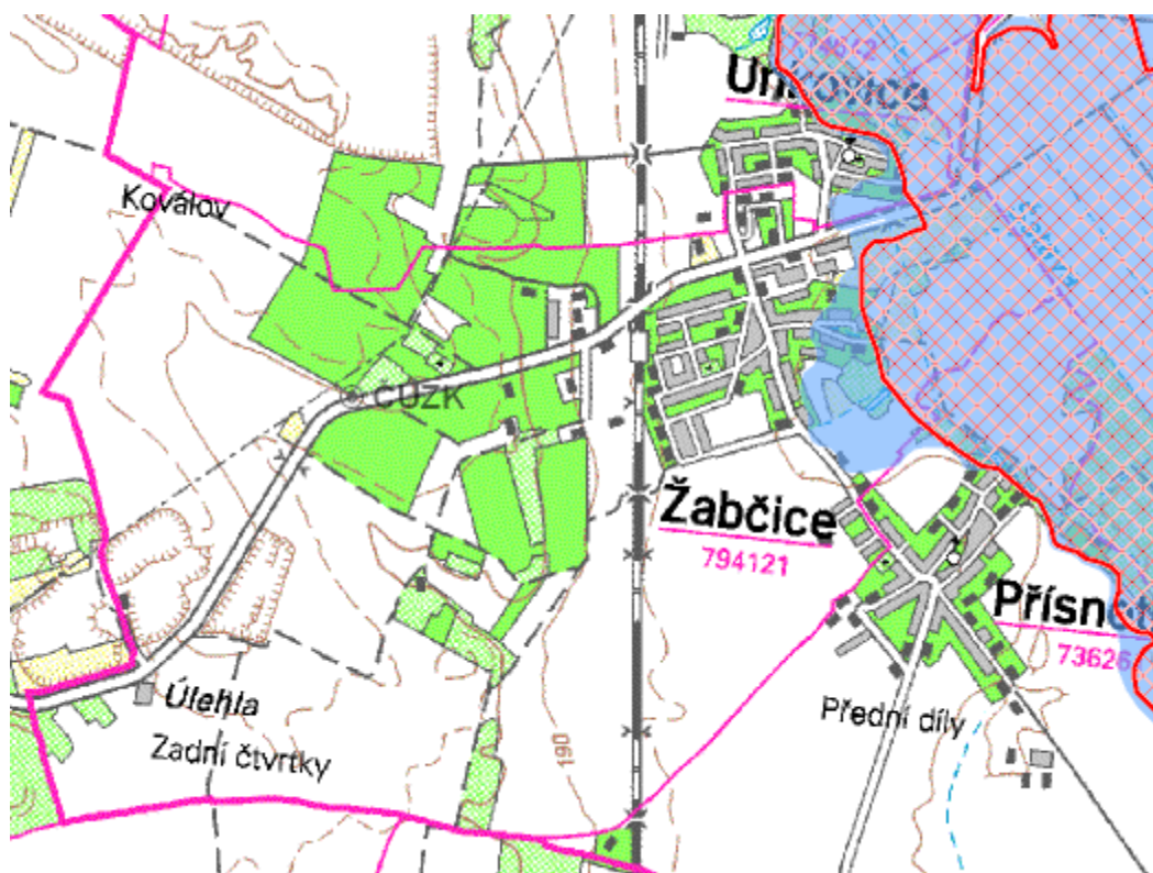
Obr. 25 Záplovové území pro průtok stoleté vody a aktivní zóna záplavového území pro Q100 v obci Žabčice.
